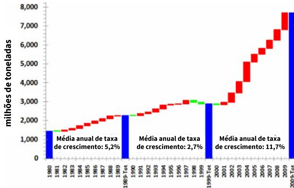
Emissões de CO 2 na China a partir de uso de energia (EIA)
